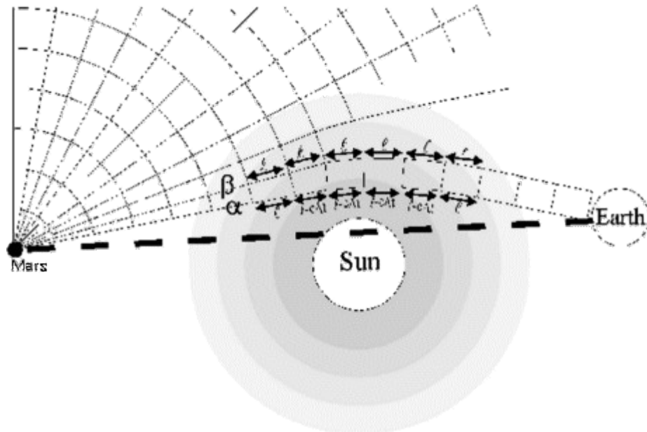
Abbildung 4: Verzögerung durch das Sonnenplasma
